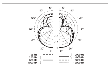
Diagrama polar (hipercardióide)
