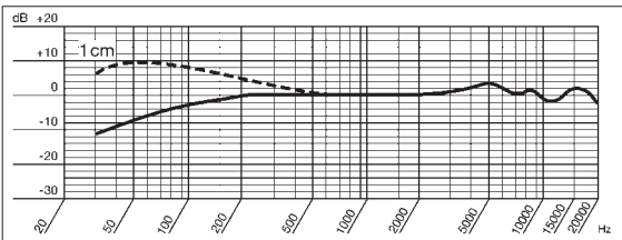
Réponse en fréquence (hypercardioïde)
