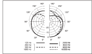
Diagramme polaire (cardioïde)
