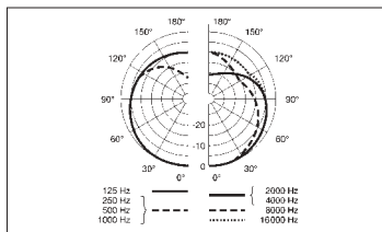
Diagrama polar (cardióide)
