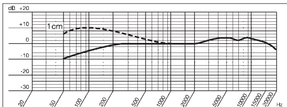
Resposta de frequência (cardióide)
