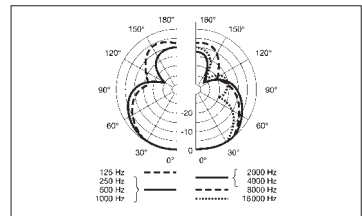
Diagramme polaire (hypercardioïde)
