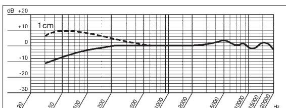
Resposta de frequência (hipercardióide)
