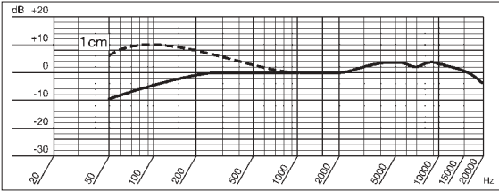
Réponse en fréquence (cardioïde)
